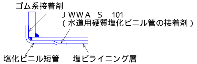
(2) 重ね合わせ接着法
