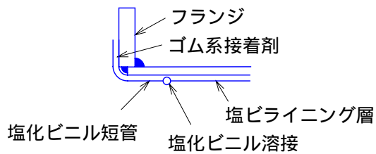
(1) 突き合わせ溶接法
