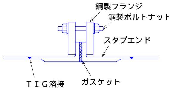
(1) スタブエンドを使用したフランジ接合の場合 (管端つば出しステンレス鋼管継手の場合も本図に準ずる)
