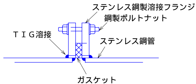
(2) 溶接フランジを使用したフランジ接合の場合
