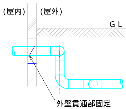
〔立面〕
