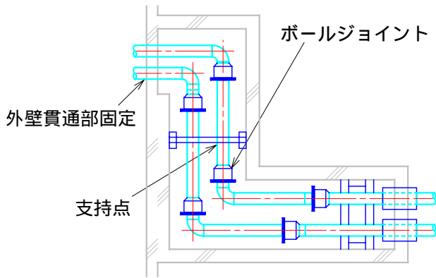
〔平面〕
