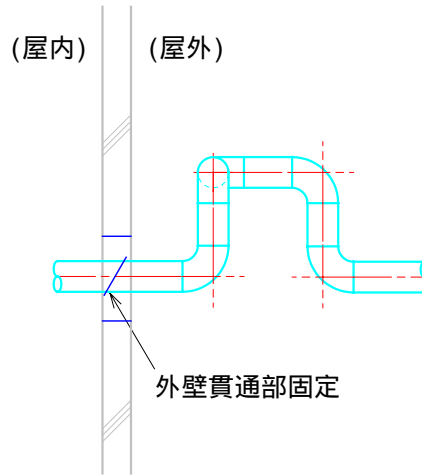
〔平面〕
