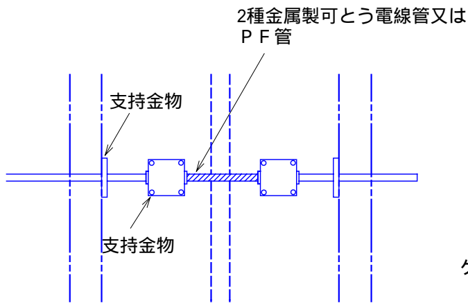
(平面)
