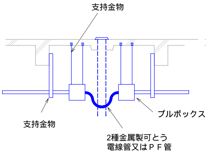
(断面)
