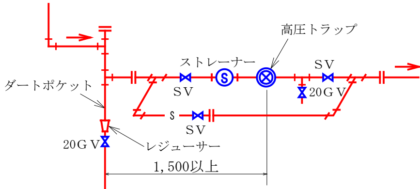
(a) 高圧トラップ装置
